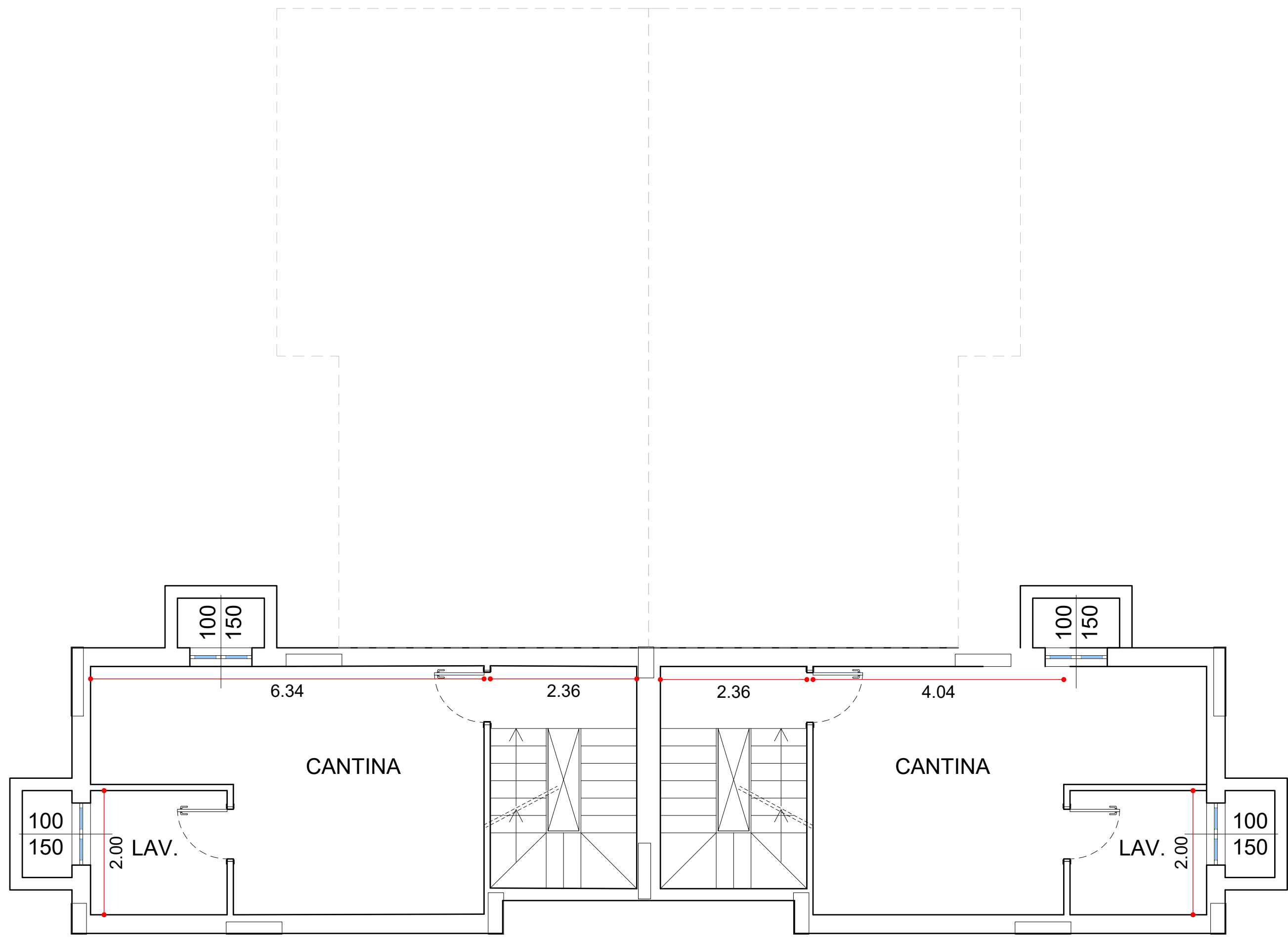
PIANTA PIANO INTERRATO
