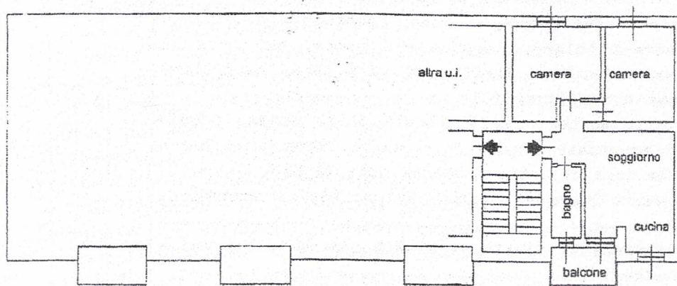
PIANO PRIMO H. 3.00 mt
